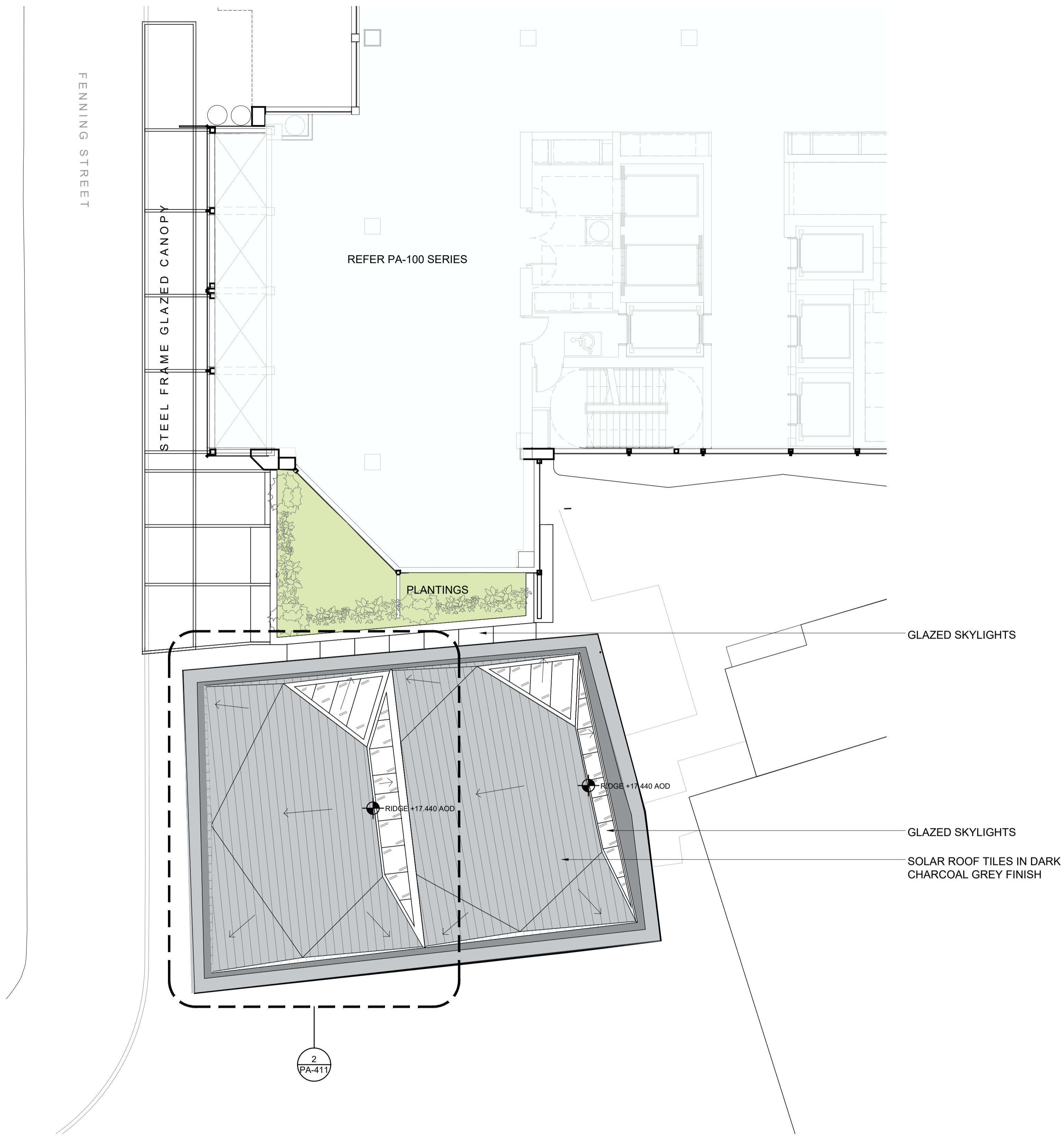
1 PLAN - ROOF SCALE: 1:100
