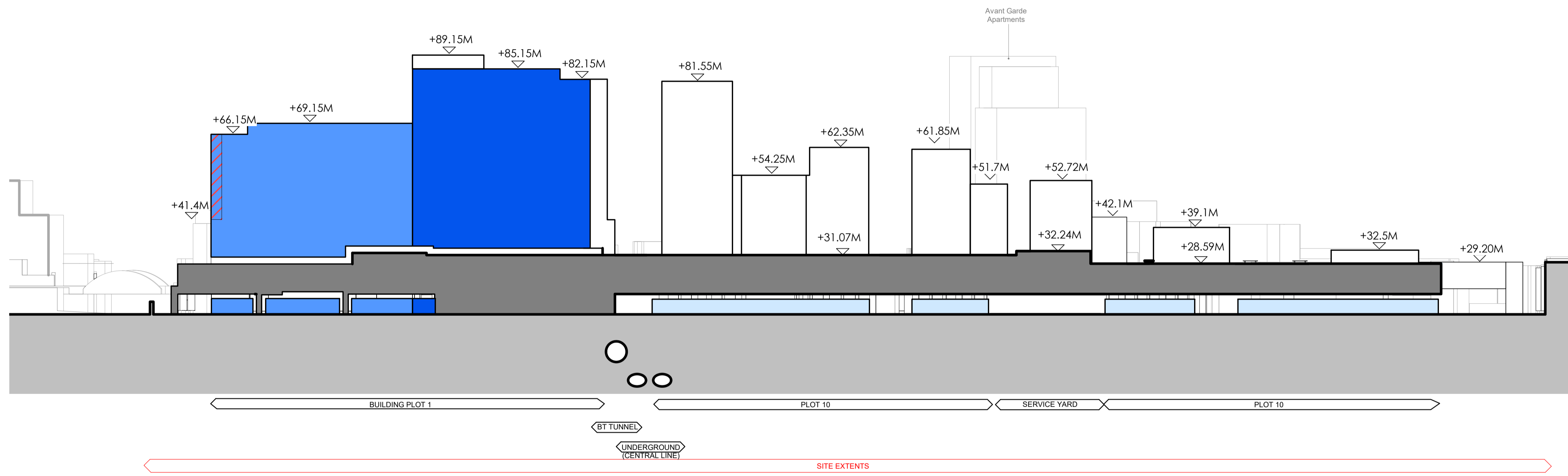
PARAMETER SECTION 1-1 1:750
