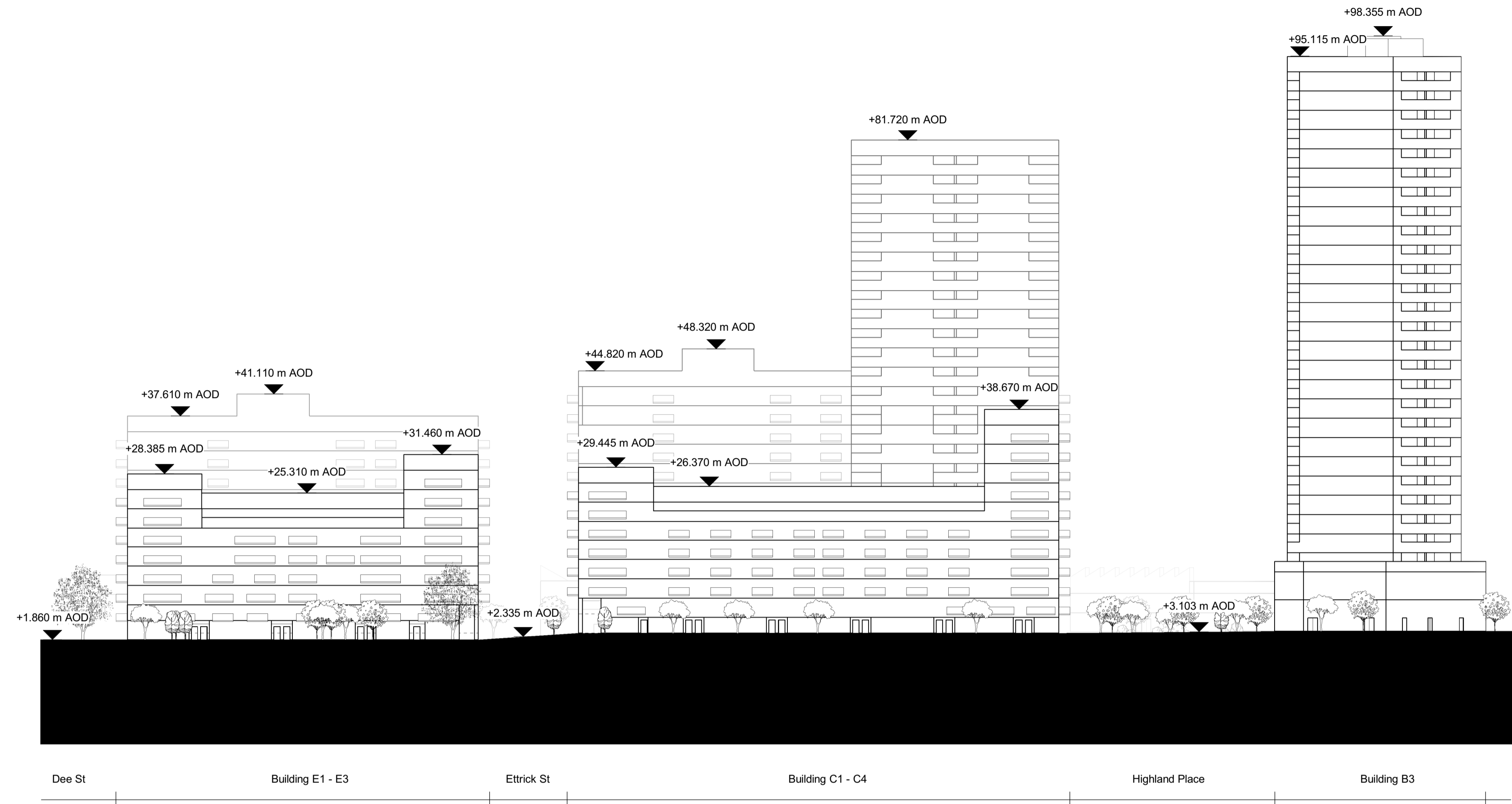
01 Elevation
