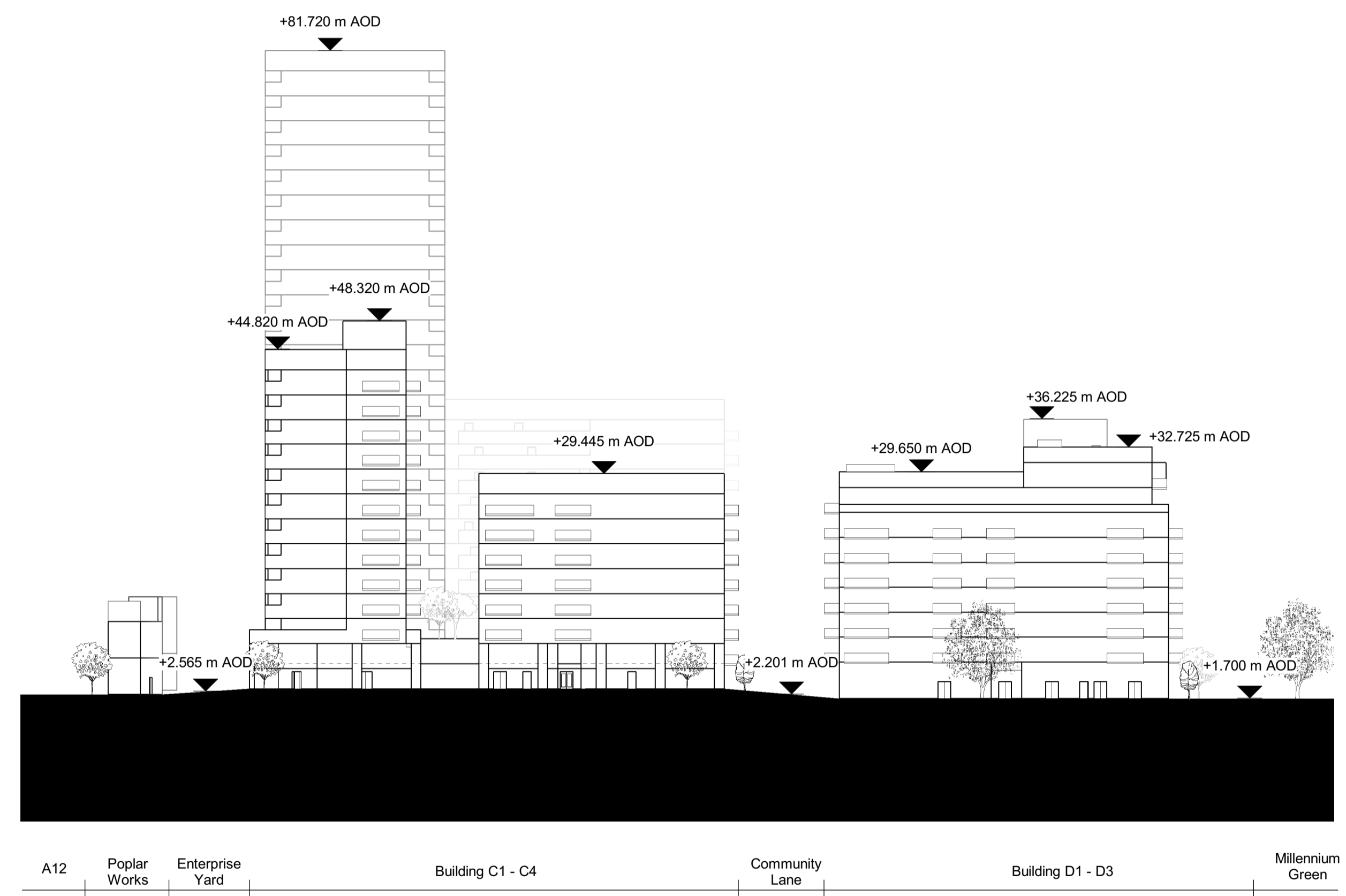
01 Elevation
