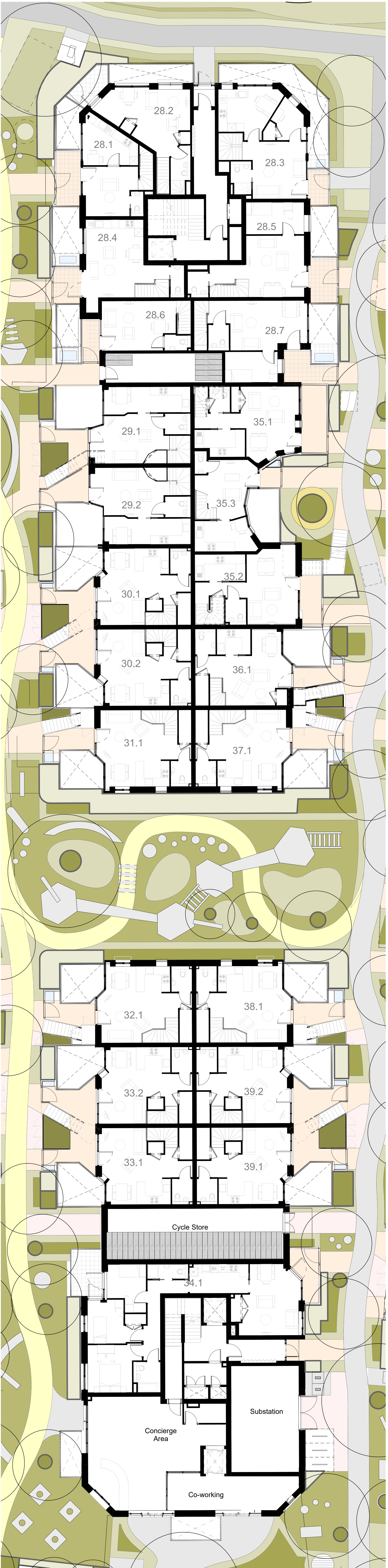
2 Block E,F - Plan GF 1 : 100
